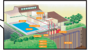
プール冷暖房給湯システム
